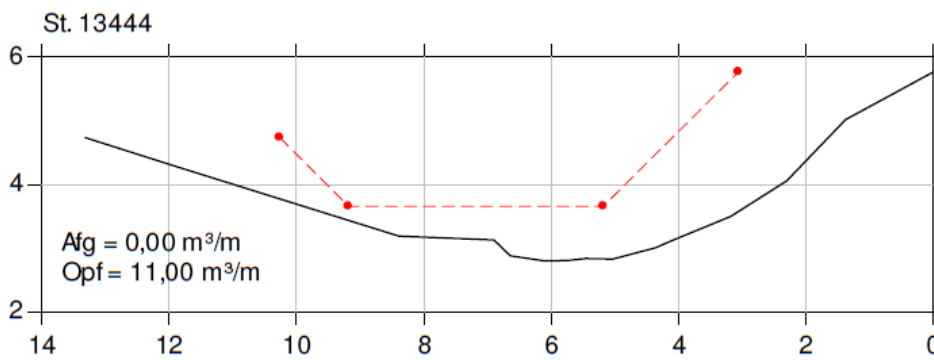
Figur 3 Opmåling fra 2009 af Køge Å station 13.444. Opmålt bundkote ligger væsentligt dybere end, der er fastsat i regulativet på ca. 2,8 DNN. Der krydses i ca. station 13.100
