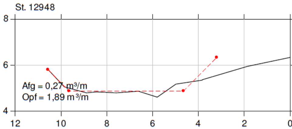
Figur 2 Opmåling fra 2009 af Køge Å station 12.948. Opmålt bundkote ligger sammenfaldende med den der er fastsat i regulativet på ca. 4,8 DNN. Der krydses i ca. station 13.100
