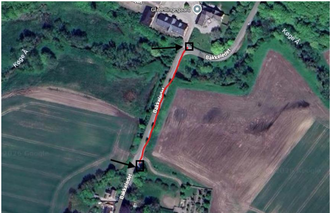
Figur 1 Viser linjeføring af kommende kabelanlæg i rød streg med pil ved afsender- og modtagegrube for underboringen.
