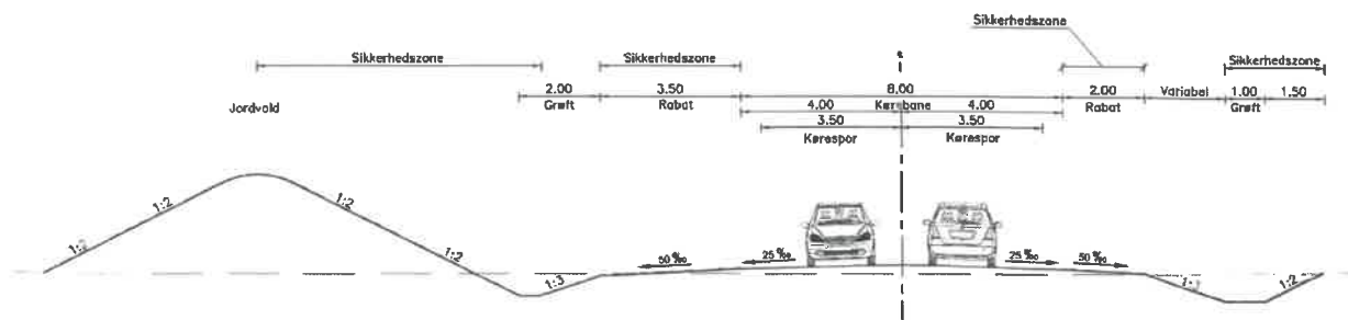
Figur 2 Normaltværprofil Adgangsvejen
