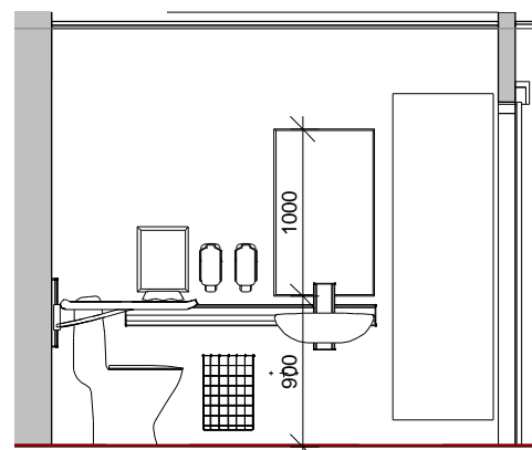
Opstalt A 1 : 50
