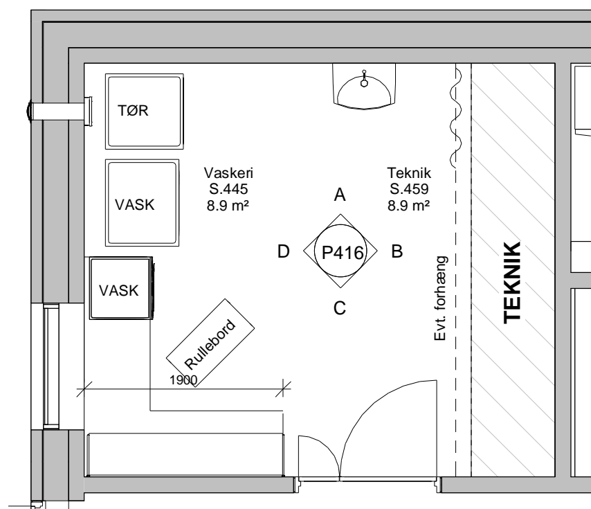
Planudsnit vaskeri / teknik 1 : 50
