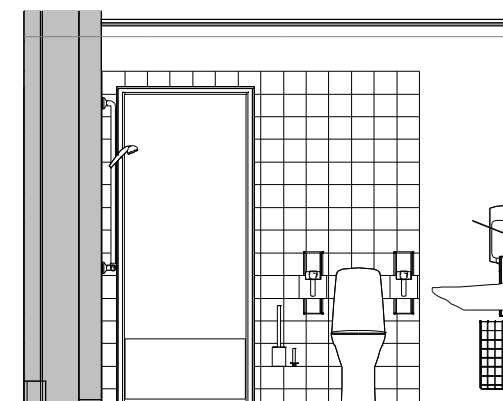
Opstalt D 1 : 50
