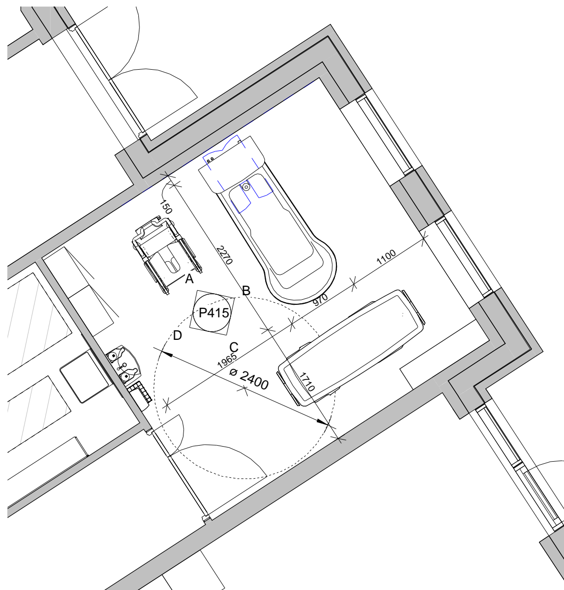
Planudsnit fællesbad 1 : 50
