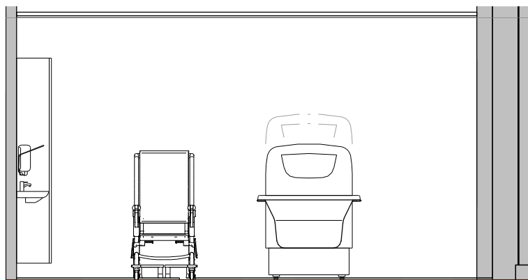
Opstalt A 1 : 50
