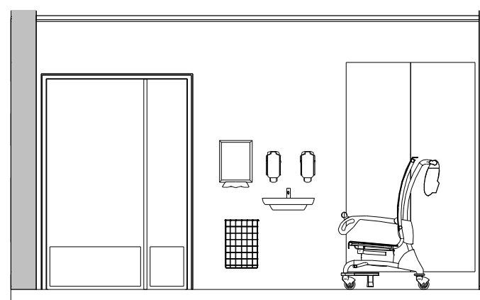
Opstalt D 1 : 50
