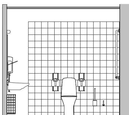
Opstalt boligtype 1 bad B 1 : 50
