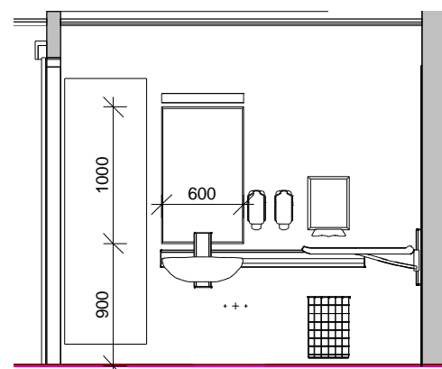
Opstalt boligtype 1 bad A 1 : 50
