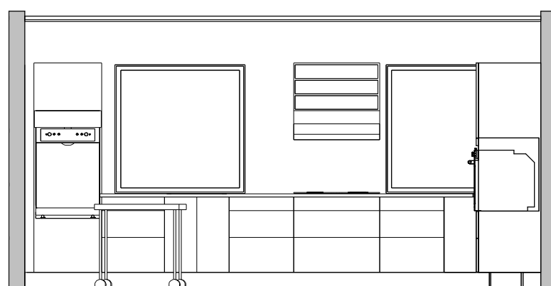
Opstalt A
