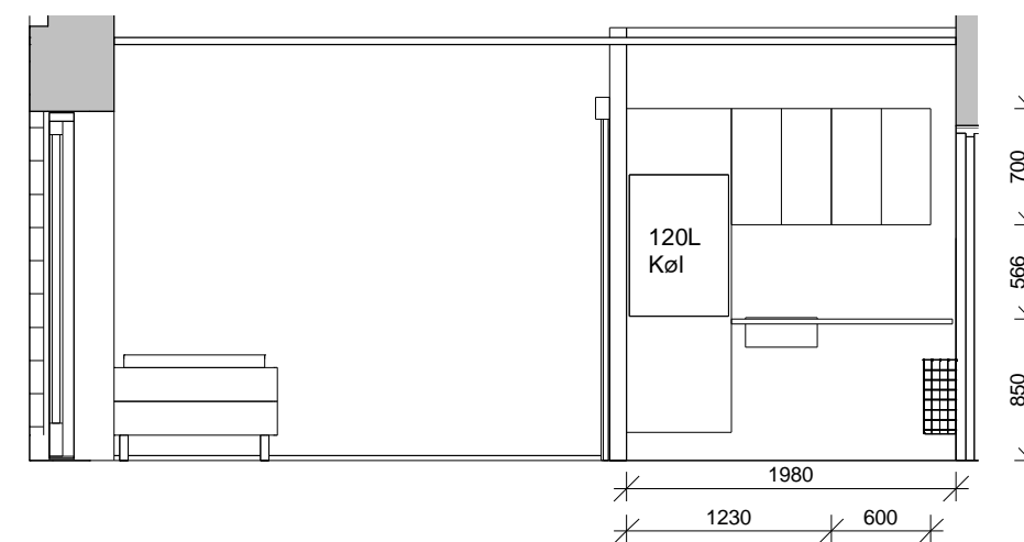
Opstalt B
