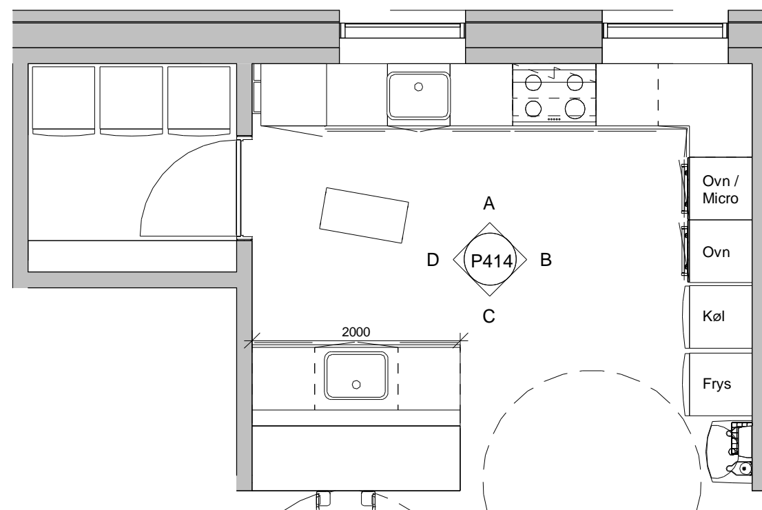
Planudsnit fælleskøkken
