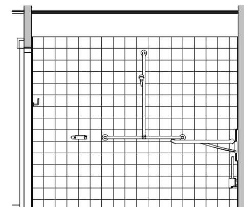
Opstalt C 1 : 50
