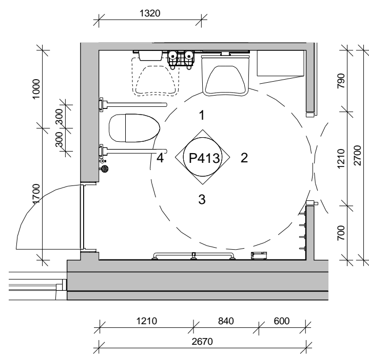
Planudsnit boligtype 2 bad 1 : 50
