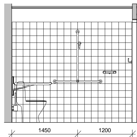
Opstalt boligtype 1 bad C 1 : 50
