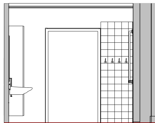
Opstalt B 1 : 50
