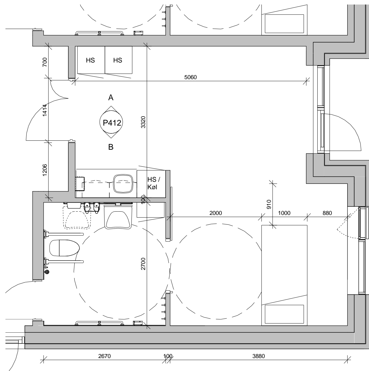
Planudsnit bolig type 2 bolig
