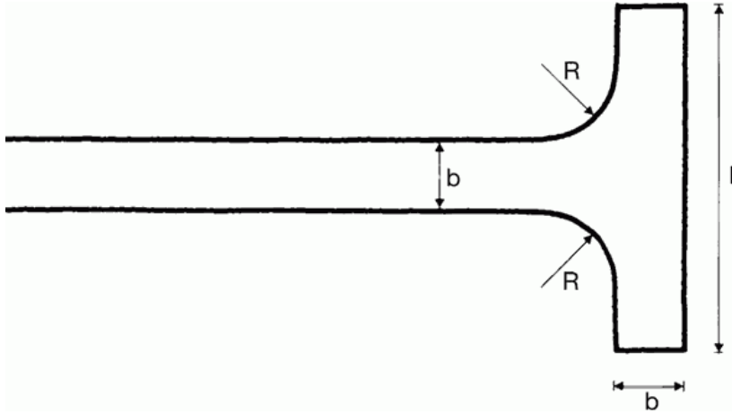
Vendeplads udformet som symmetrisk hammerhoved, principskitse
