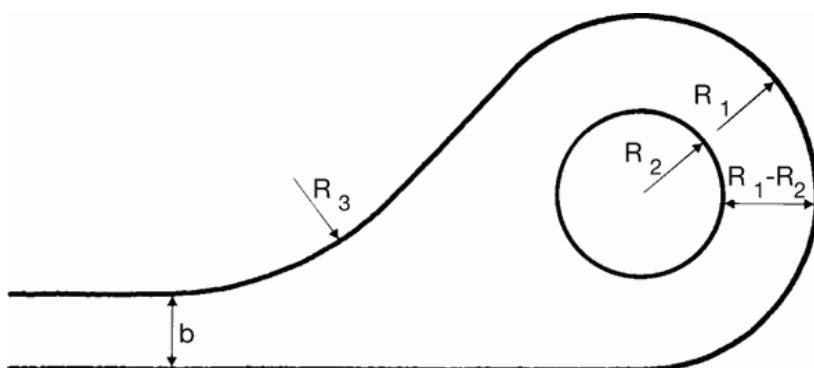
Cirkelformet vendeplads, principskitse
