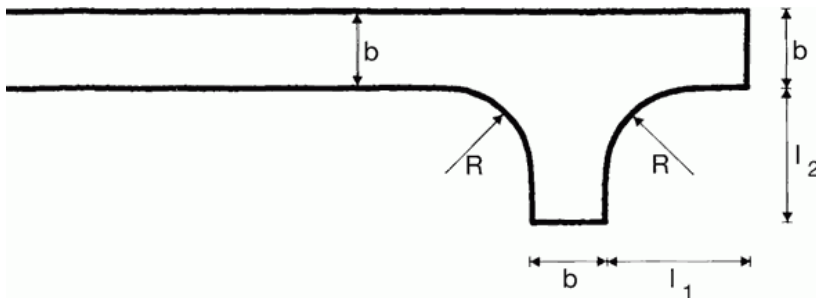
Vendeplads udformet som asymmetrisk hammerhoved, principskitse
